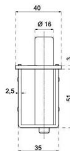
Gond à déclic rapide, partie inférieure
