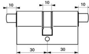
Cylindre profilé avec triangle externe
