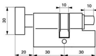
Cylindre profilé bouton avec triangle interne
