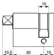
1/2 Cylindre profilé avec triangle externe
