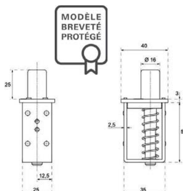
Gond à déclic rapide, partie supérieure
