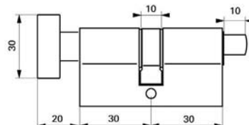
Cylindre profilé bouton avec triangle externe
