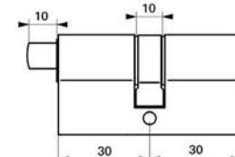
Cylindre profilé avec triangle externe
