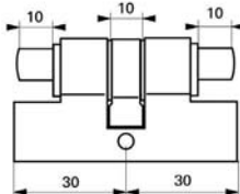
Cylindre profilé avec triangle interne
