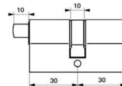
Cylindre profilé avec triangle externe
