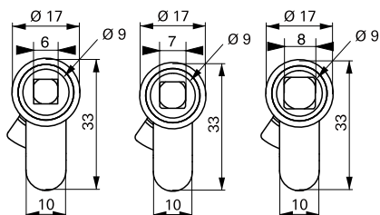
1/2 Cylindre profilé avec triangle externe
