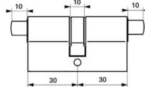
Cylindre profilé avec triangle externe
