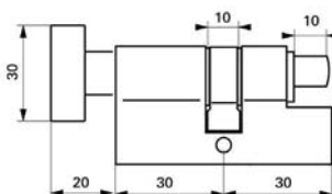
Cylindre profilé bouton avec triangle interne
